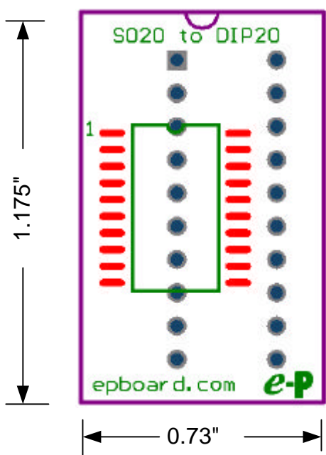
Top Side
