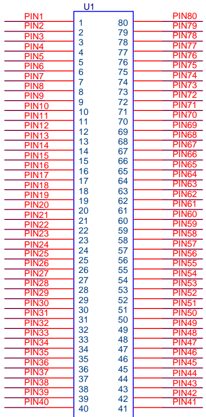
TQFP80
